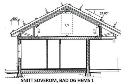
SNITT SOVEROM, BAD OG HEMS 1
