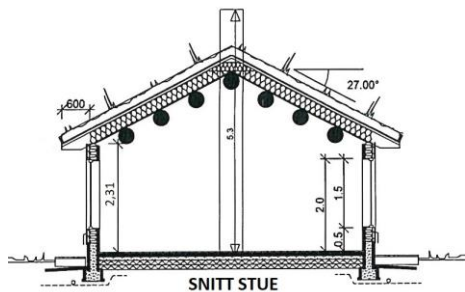
SNITT STUE
